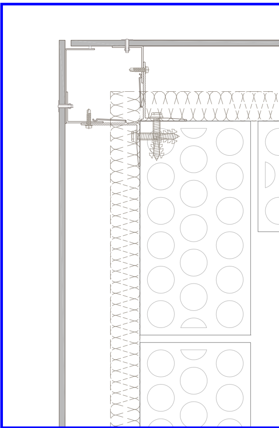
ESQUINA EXTERIOR
