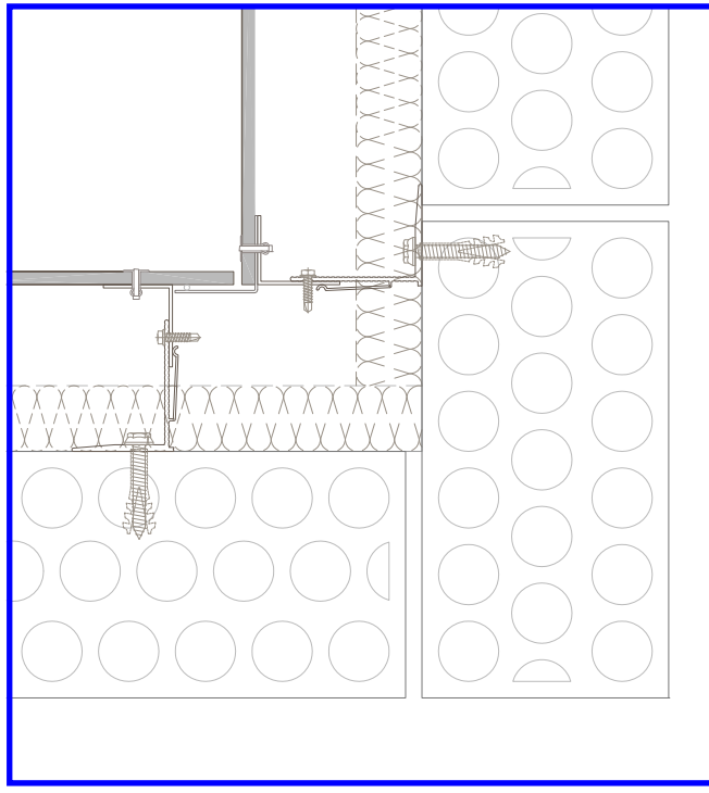
ESQUINA INTERIOR
